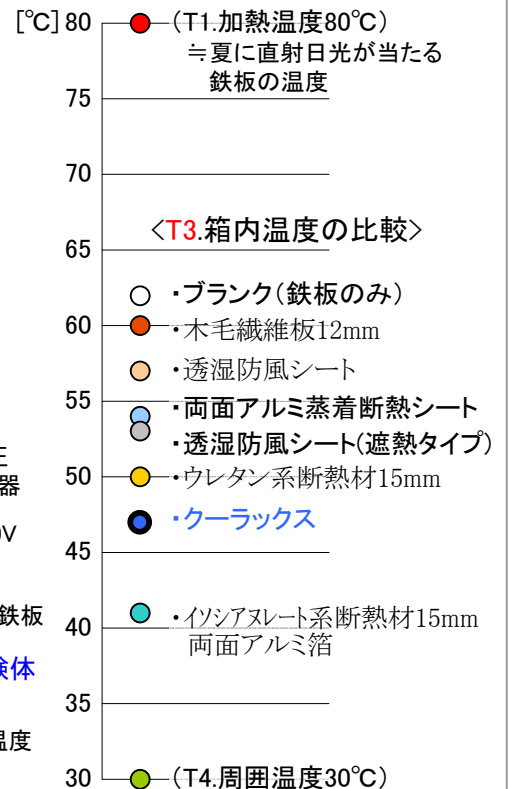
—表面材による箱内温度の比較—
