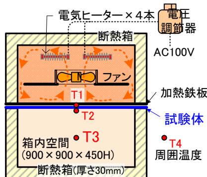
—屋内実験装置—
